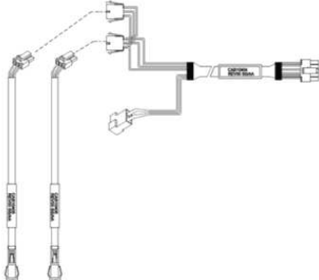
Electrical Cables (Ref.: PRD10521)
