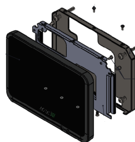
Suporte mecânico fixo parede (Ref. PRD10706) *
