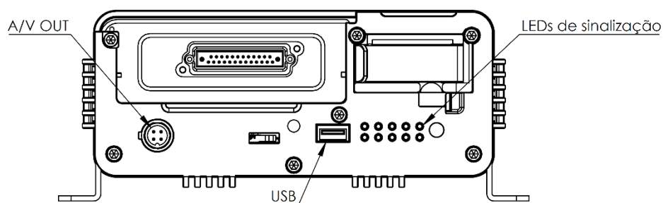
Parte Traseira
