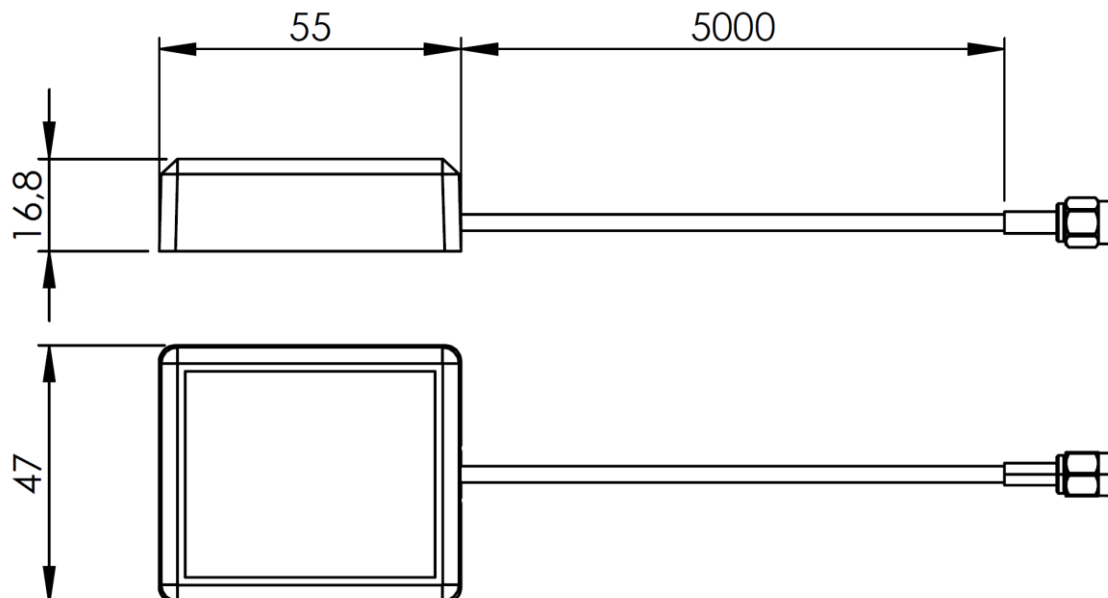
Antena GPS
