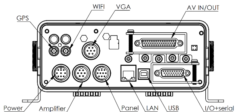
Parte Traseira
