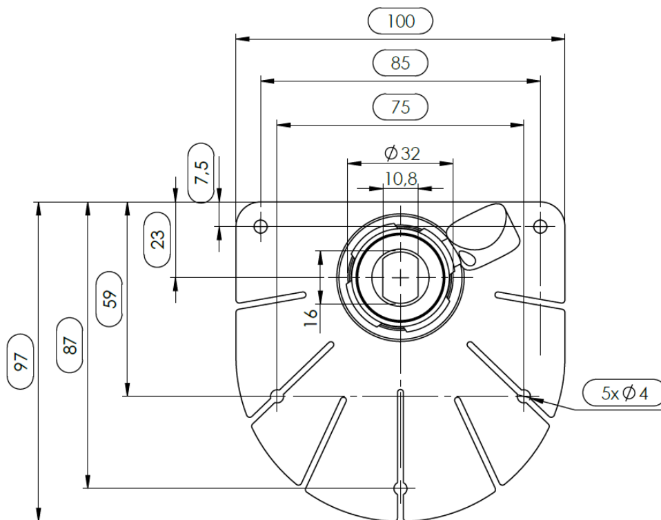
Vista Superior Suporte Articulado
